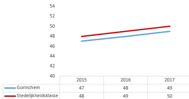
Duurzaamheidsscore
